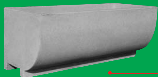
mod. 71/100 cm 100x42xH40 peso kg 128 incastro cm 16,5 per balconi
