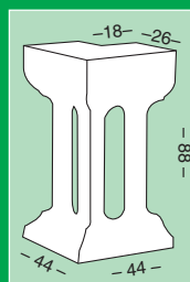
mod. 13 cm 44x44xH88 peso kg 68
