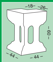
mod. 11 cm 44x44xH60 peso kg 62
